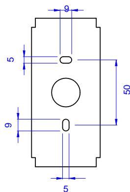
PLAQUE DE MONTAGE
