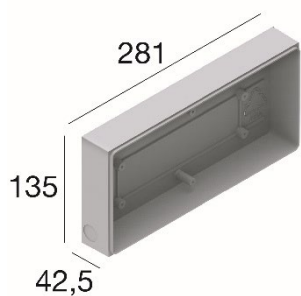
Boîtier d'installation 281 x 135 x 42.5 mm
