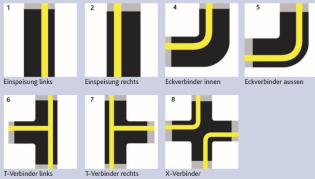
Einspeisung links und Einspeisung rechts
